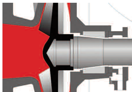
KONISCHE STOPFBUCHSE
